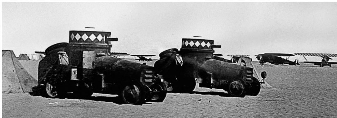
Ιταλικά τεθωρακισμένα οχήματα και αεροσκάφη που συμμετείχαν στην κατάληψη της Κούφρα στις 20 Ιανουαρίου 1931.
