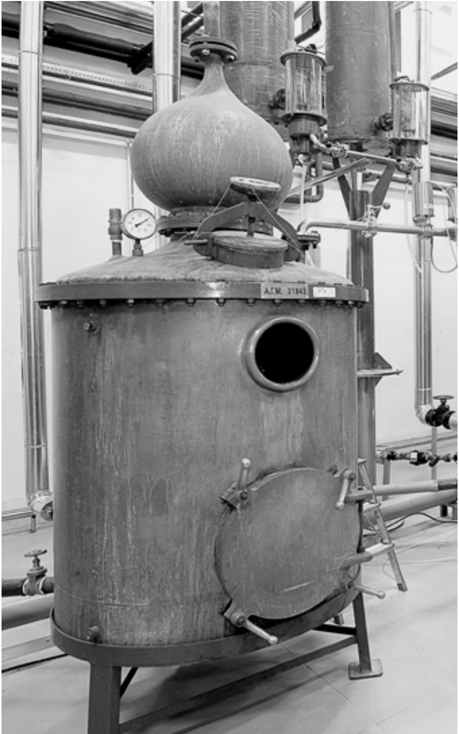
Άμβυκας απόσταξης ούζου. ΑΠΕΝΑΝΤΙ: Το ουζερί «Τσινάρη», στην Άνω Πόλη της Θεσσαλονίκης, λειτουργεί από το 1885.
